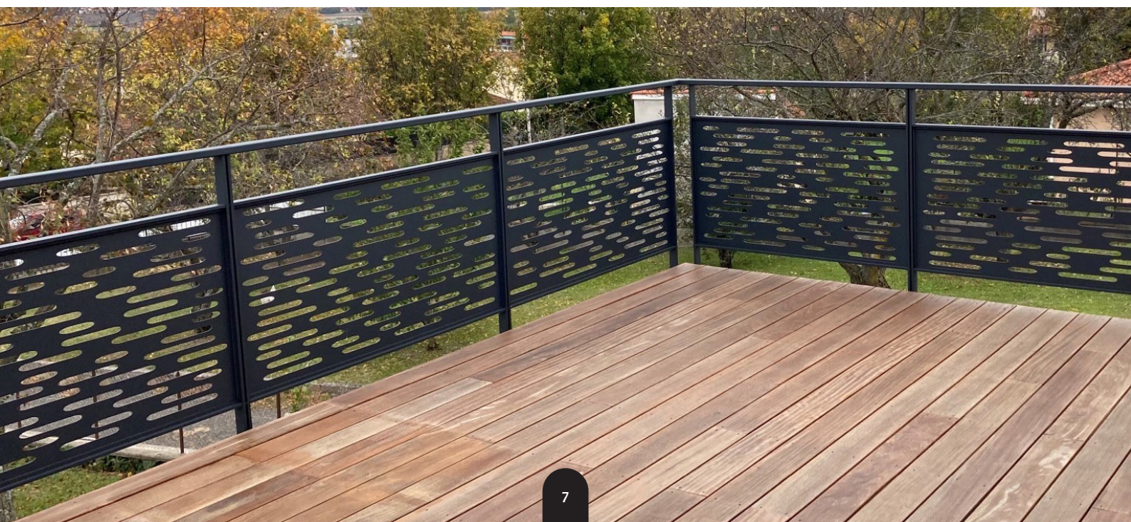
Tôle perforée axée / 2 espaces sous main-courante / Fixation à plat Montants espacés
